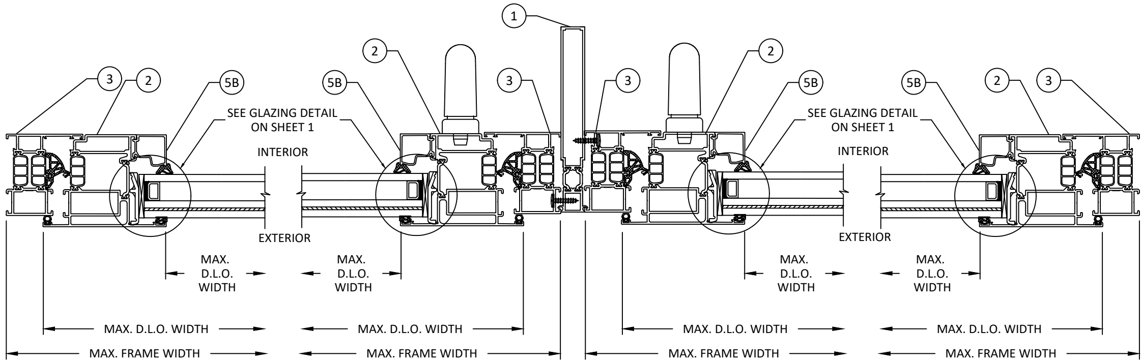
A HORIZONTAL SECTION 5 TYP. JAMB DETAIL
