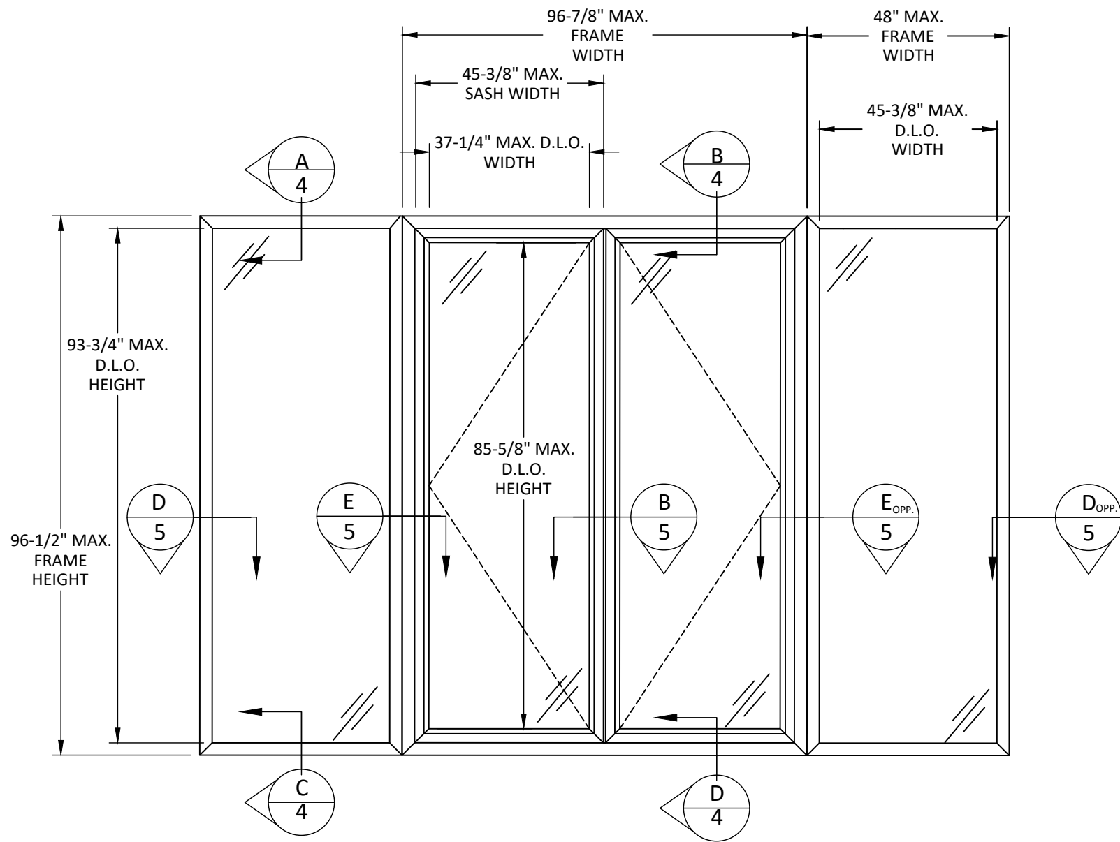
ELEVATION
