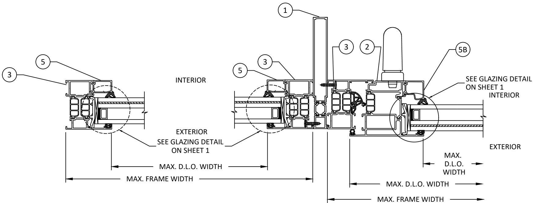
A HORIZONTAL SECTION 5 TYP. JAMB DETAIL
